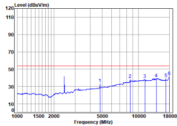
BLE_2M_TX_CH_19_Horizontal-Avg
