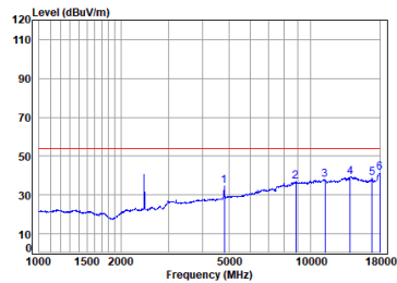
BLE_2M_TX_CH_19_Vertical-Avg
