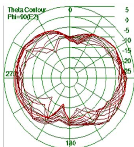
2500 MHz E2
