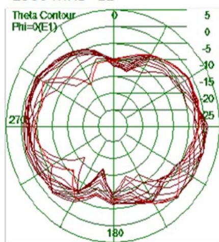
2500 MHz E1
