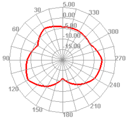
2480.000MHz E1
