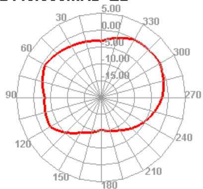
2440.000MHz E2
