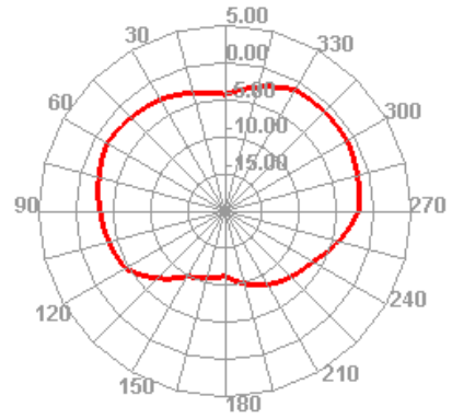
2480.000MHz E2
