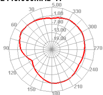
2440.000MHz H
