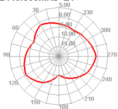
2440.000MHz E1
