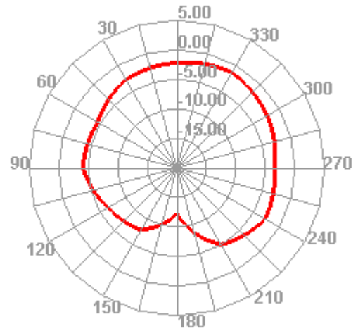
2480.000MHz E2
