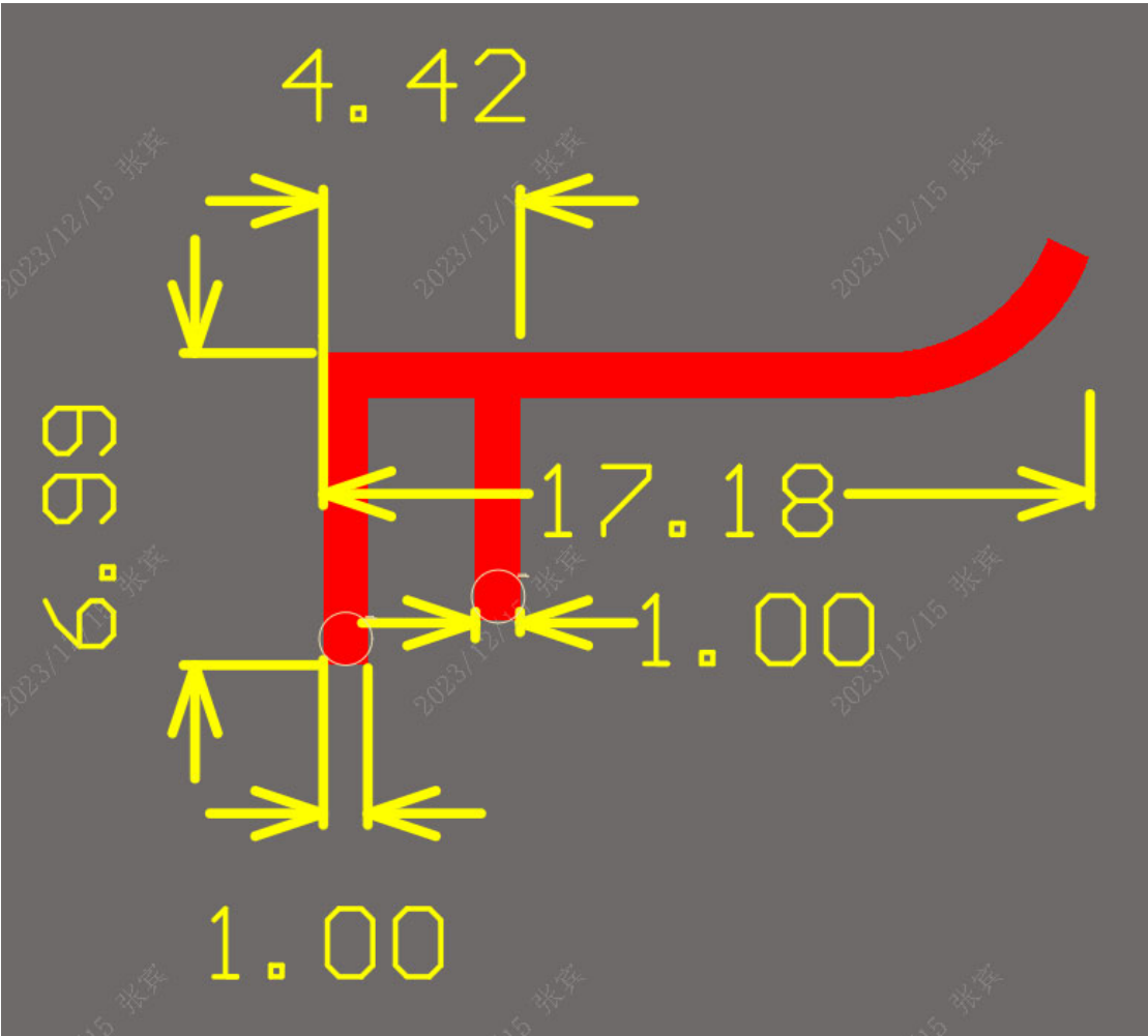
天线尺寸 (单位: mm)
