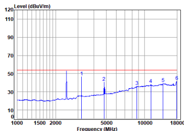
11g_TX_CH_06_Horizontal-Avg
