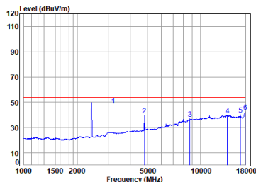
11g_TX_CH_01_Horizontal-Avg
