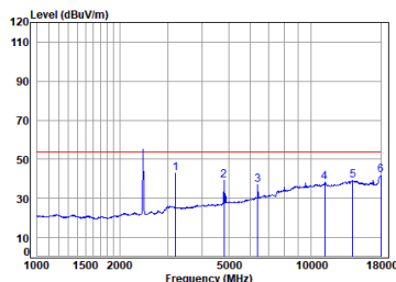
11g_TX_CH_06_Vertical-Avg
