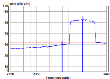
11ax_40M_TX_CH_03_Horizontal-Avg
