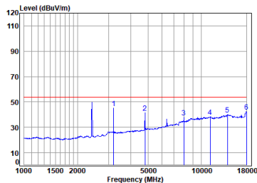
11g_TX_CH_01_Vertical-Avg
