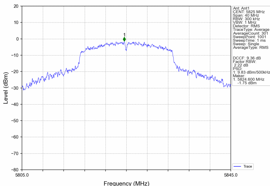
802.11n(HT20)_HCH_5825MHz_Ant1_NTNV
