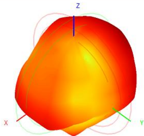
远场方向图
