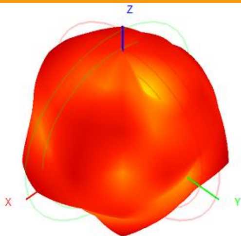
远场方向图
