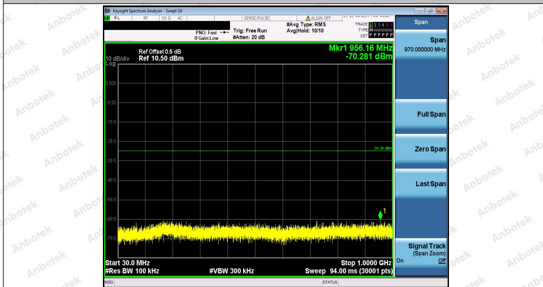
2.4G_Ant1_2441_30~1000
