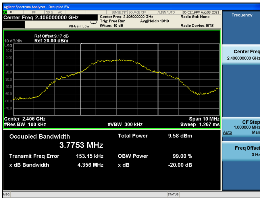
2406MHz
