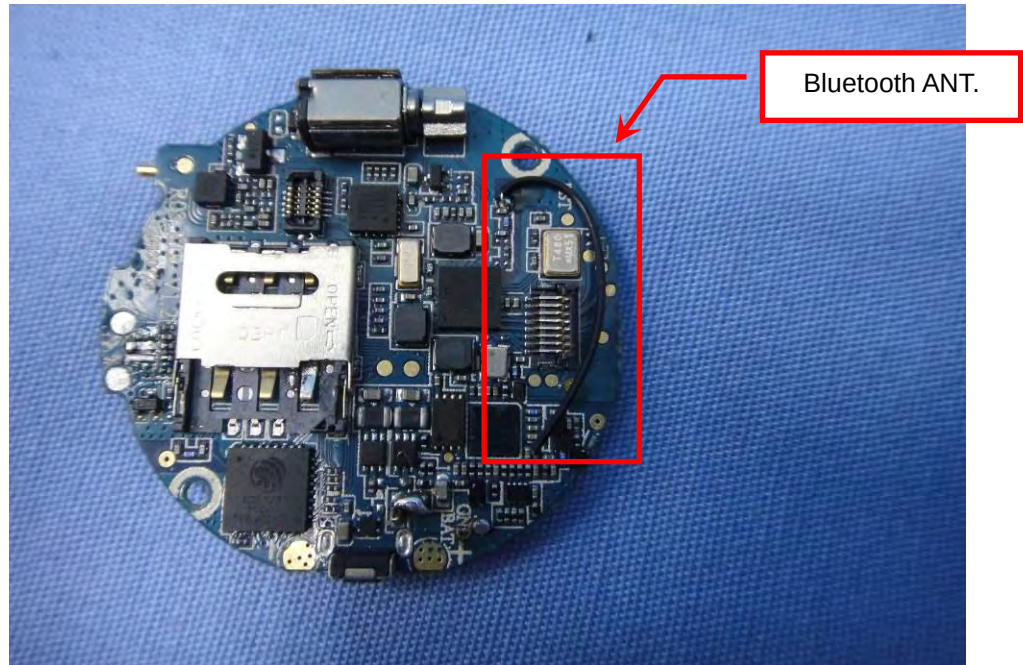
EUT Photo (14)
