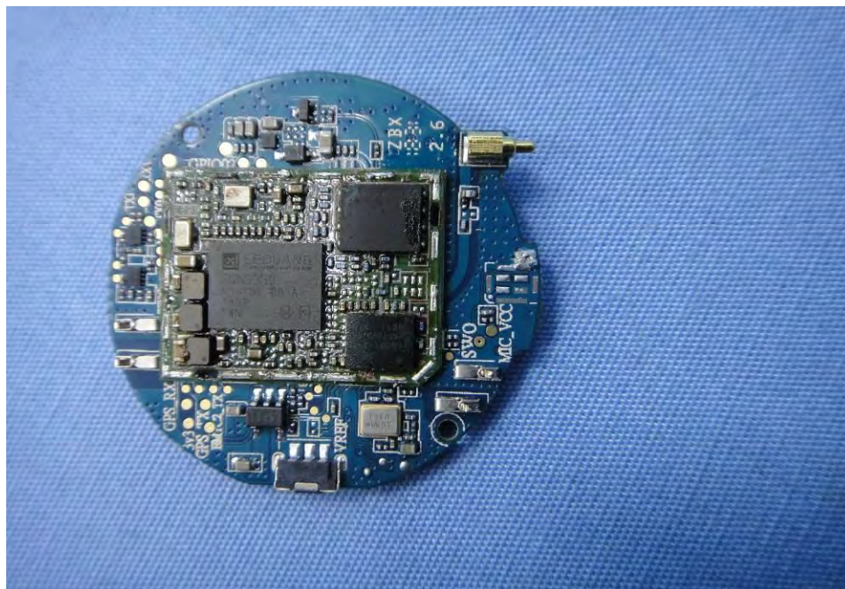
EUT Photo (15)
