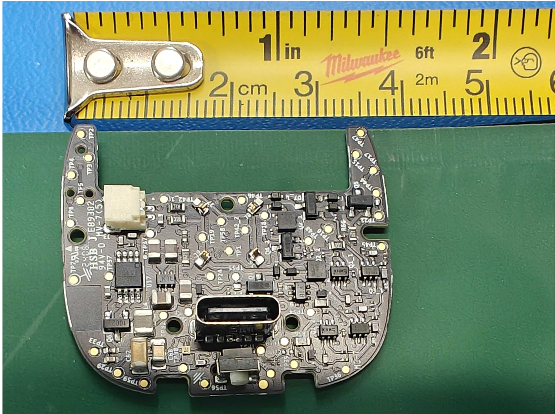
Enso 3 Device PCBA, Bottom
