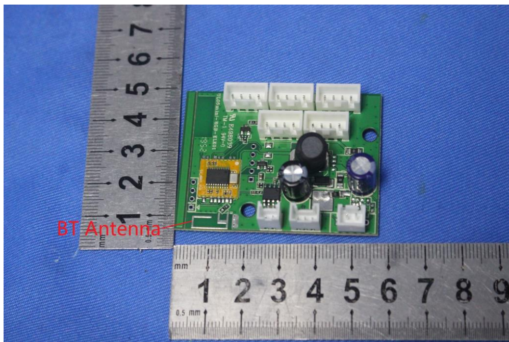
BLE Antenna
