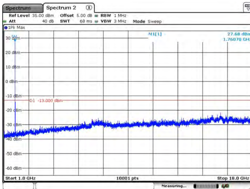
B66_CH132572_20M_1RB0_QPSK_Above 1G
