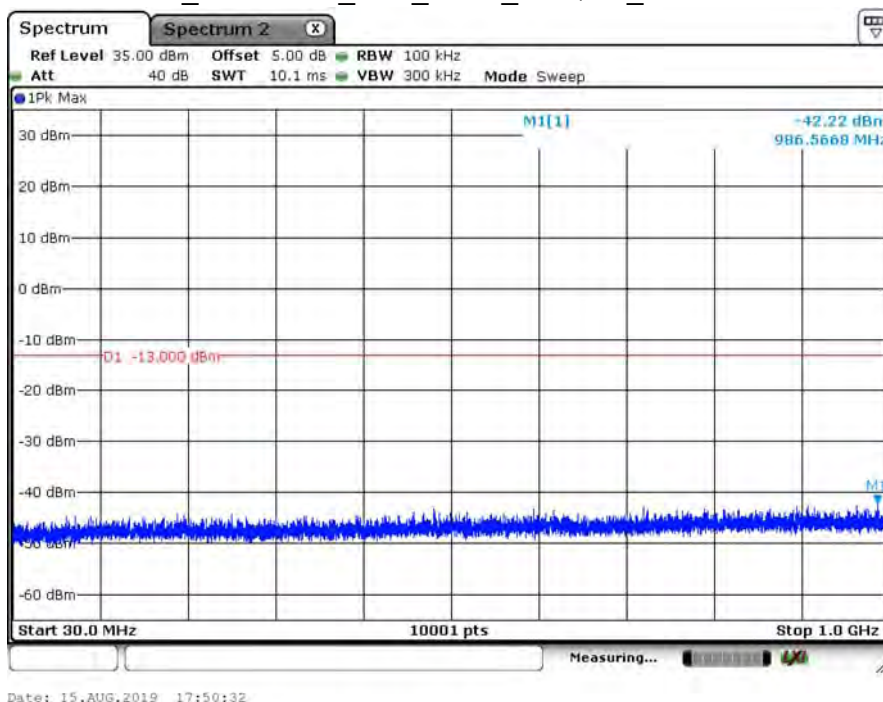
B66_CH132072_20M_1RB0_16-QAM_Below 1G
