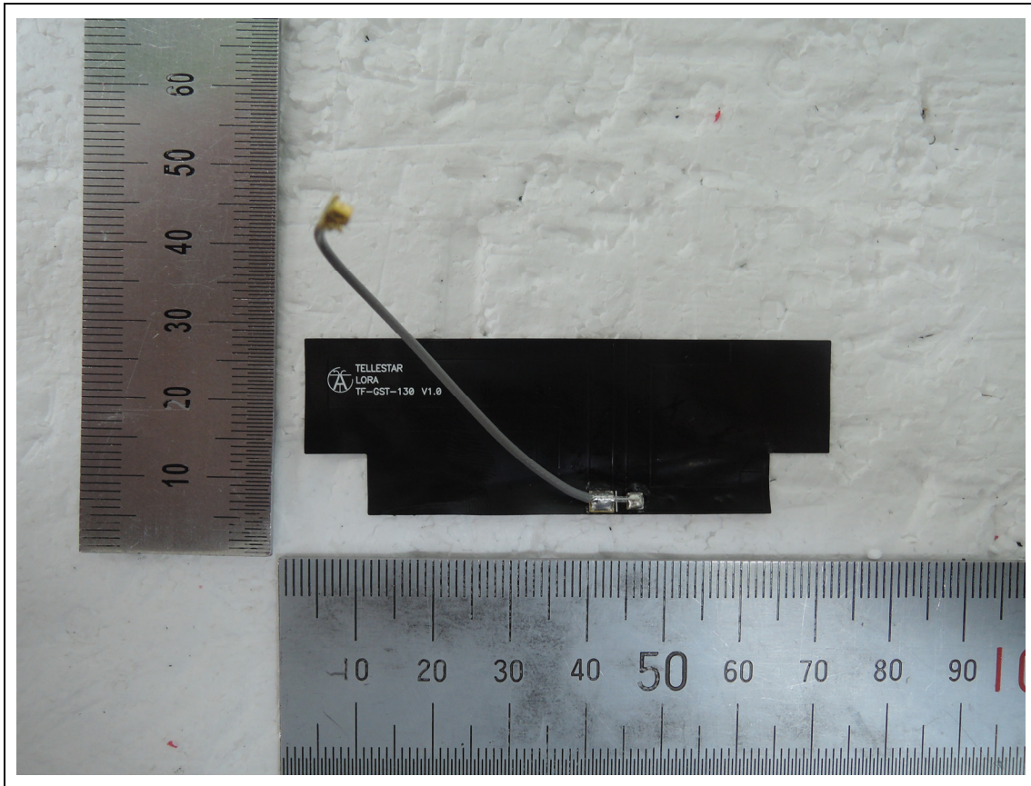
<GSM Antenna>
