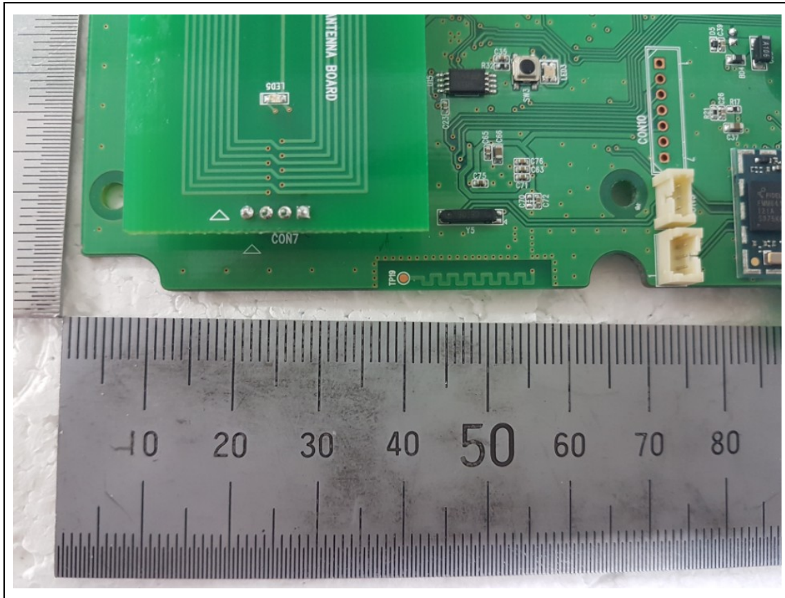
<BLE Antenna>
