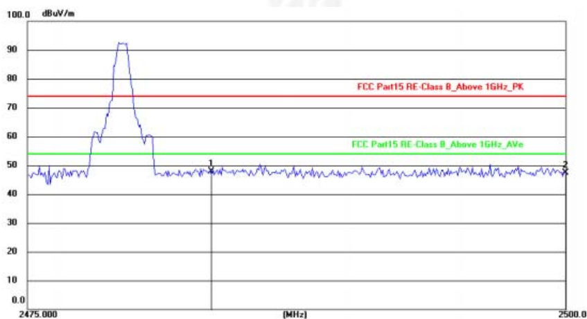
2480MHz Horizontal
