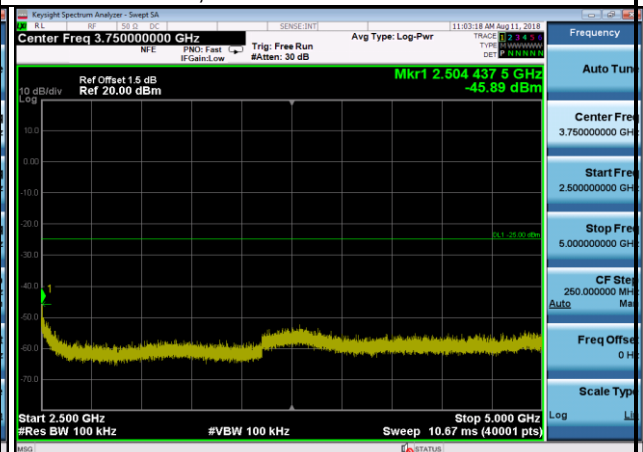
802.11n(HT20),2462MHz,Ant0,Plot 4,2500MHz~5000MHz
