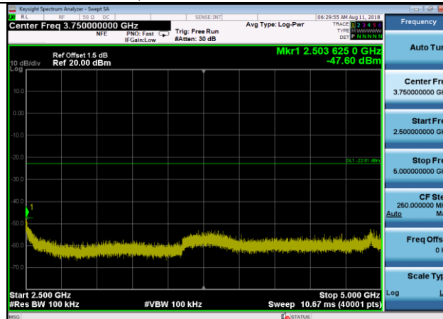
802.11n(HT20),2462MHz,Ant1,Plot 4,2500MHz~5000MHz
