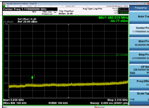
802.11g,2462MHz,Ant0,Plot 3,30MHz~2310MHz
