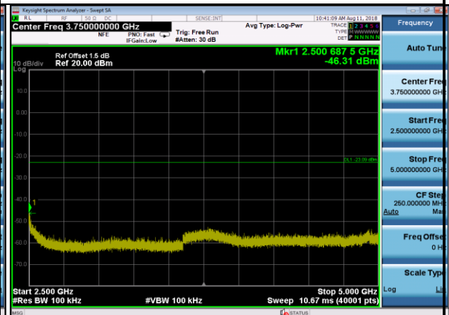
802.11g,2462MHz,Ant0,Plot 4,2500MHz~5000MHz
