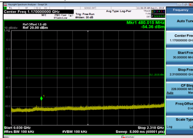
802.11n(HT40),2452MHz,Ant0,Plot 3,30MHz~2310MHz
