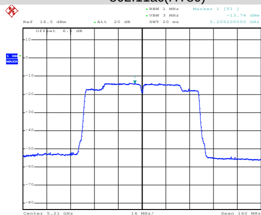
802.11ac(HT80)
