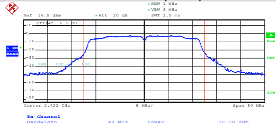
802.11n(HT40)
