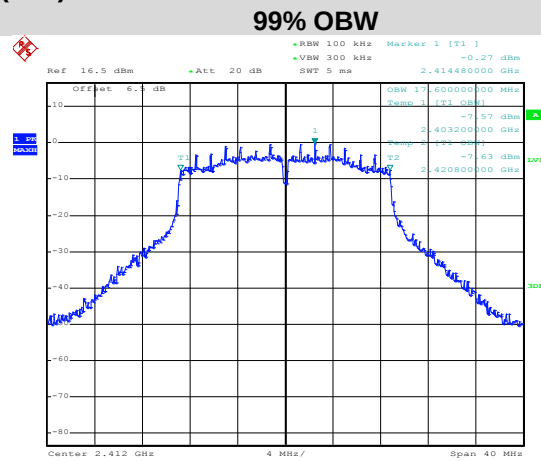
802.11n(H20)
