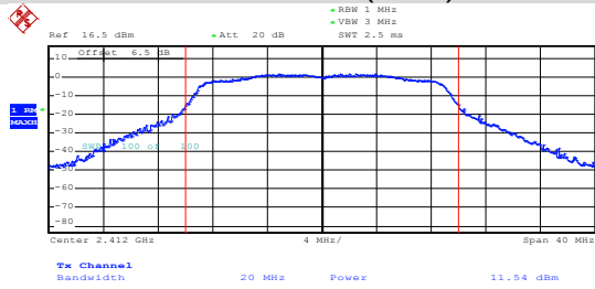
802.11n(HT20)
