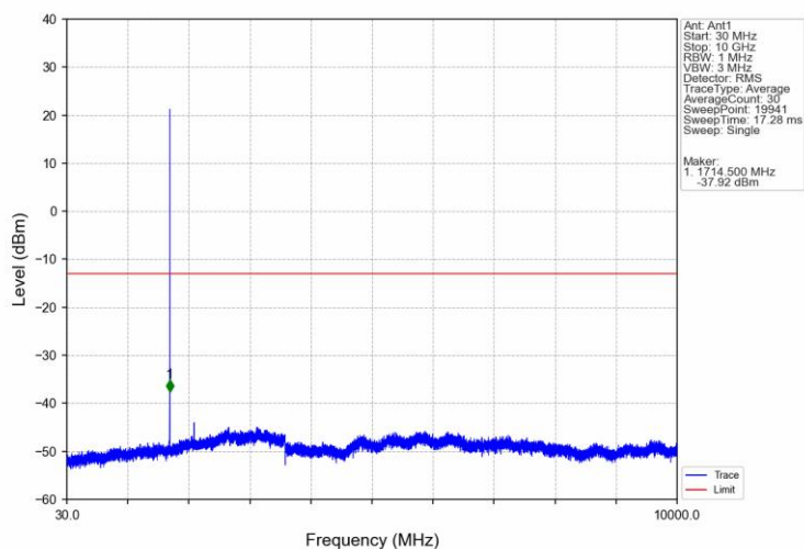
Band66 1.4MHz QPSK LCH 1710.7MHz RB 1 0 NTNV
