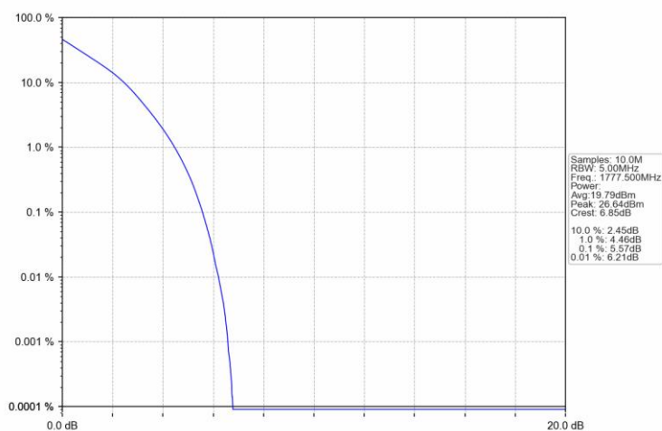
Band66 5MHz QPSK HCH 1777.5MHz RB 25 0 NTV
