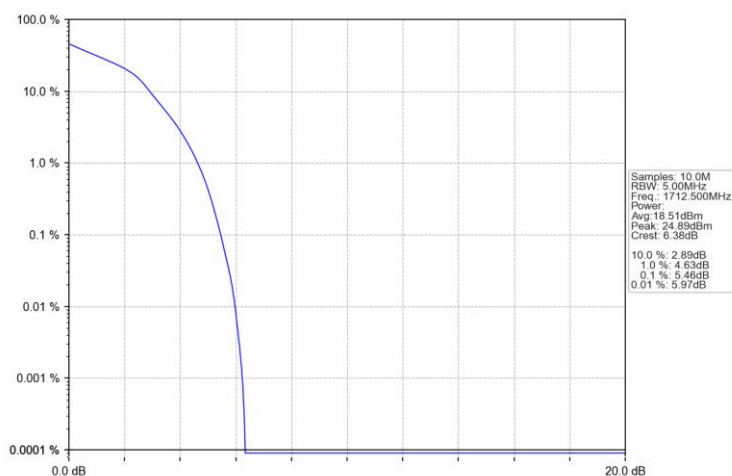
Band66 5MHz 16QAM LCH 1712.5MHz RB 25 0 NTV
