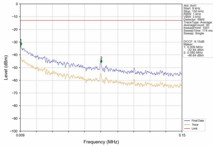
PCS1900_EGPRS_HCH_1909.8MHz_1 TX Slot_NTNV
