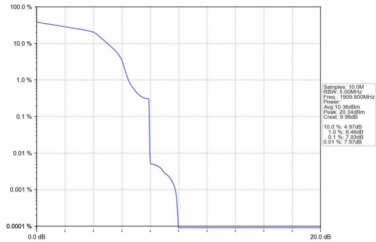
PCS1900_EGPRS_HCH_1909.8MHz_4 TX Slots_NTNV
