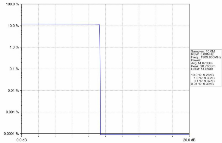
PCS1900_GSM_HCH_1909.8MHz_GSM_NTNV
