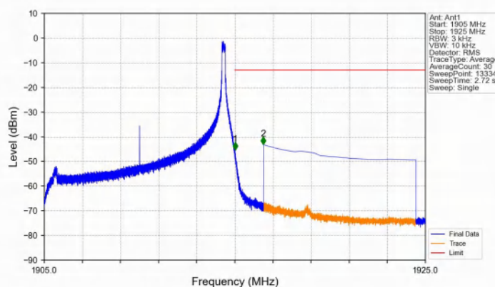
Band25_10MHz_QPSK_HCH_1910MHz_RB_1_49_NTNV
