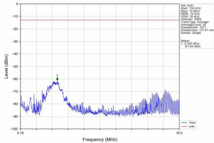
Band25_10MHz_QPSK_LCH_1855MHz_RB_1_0_NTNV
