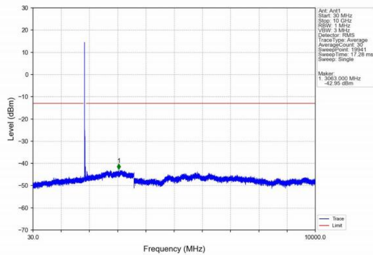
Band25_20MHz_QPSK_LCH_1860MHz_RB_1_0_NTNV
