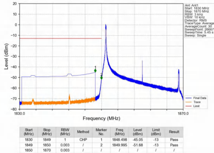
Band25_20MHz_QPSK_LCH_1860MHz_RB_1_0_NTNV
