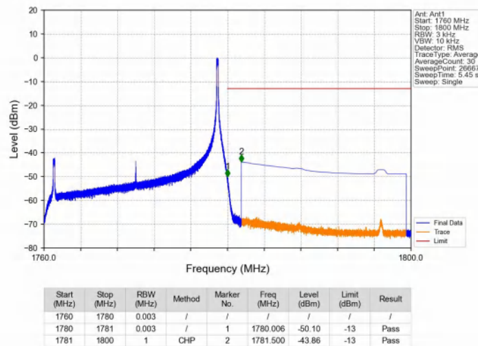
Band66_20MHz_QPSK_HCH_1770MHz_RB_1_99_NTNV
