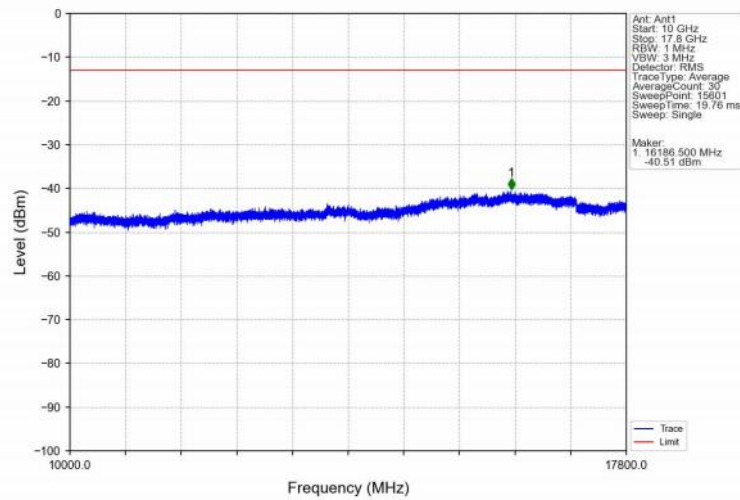
Band66_10MHz_QPSK_HCH_1775MHz_RB_1_49_NTNV
