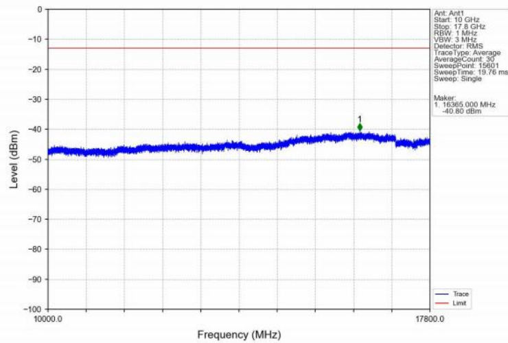
Band66_5MHz_QPSK_HCH_1777.5MHz_RB_1_24_NTNV
