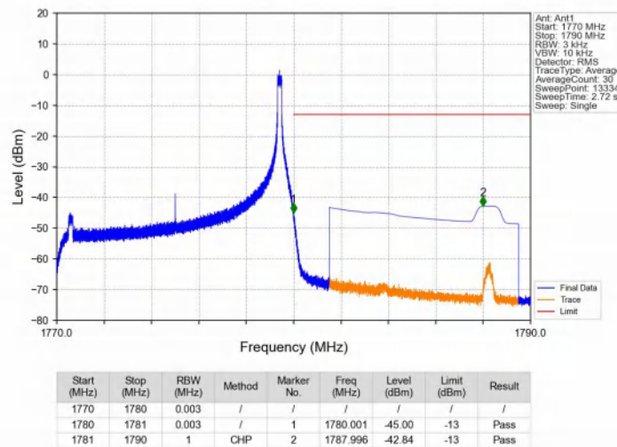
Band66_10MHz_QPSK_HCH_1775MHz_RB_1_49_NTNV
