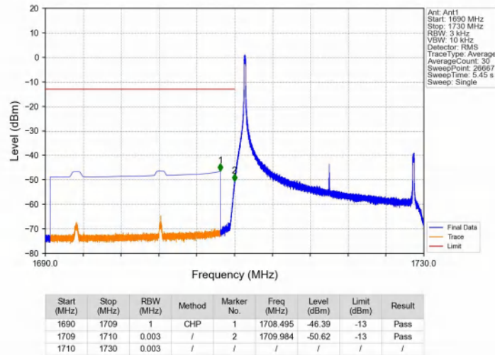
Band66_20MHz_QPSK_LCH_1720MHz_RB_1_0_NTNV
