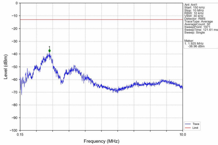
Band4_HSUPA_LCH_1712.4MHz_Subtest 1_NTNV
