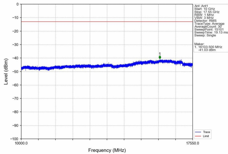
Band4_HSUPA_LCH_1712.4MHz_Subtest 1_NTNV
