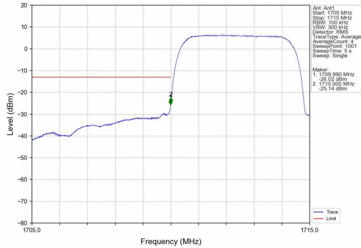
Band4_HSUPA_LCH_1712.4MHz_Subtest 1_NTNV
