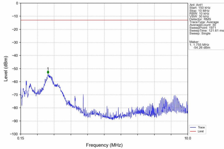
Band5_HSUPA_MCH_836.6MHz_Subtest 1_NTNV
