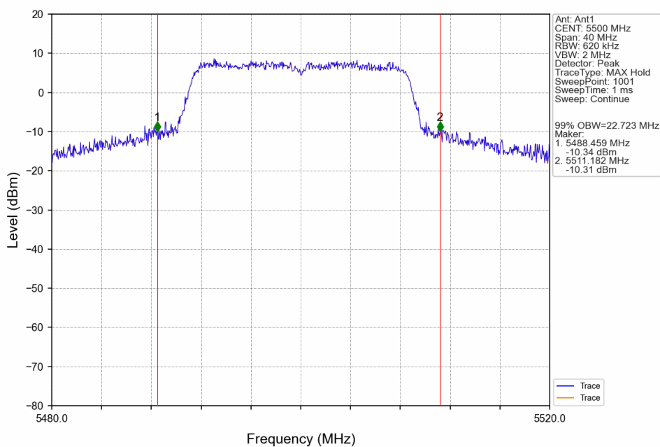
802.11ac(VHT20)_LCH_5500MHz_Ant1_NTNV
