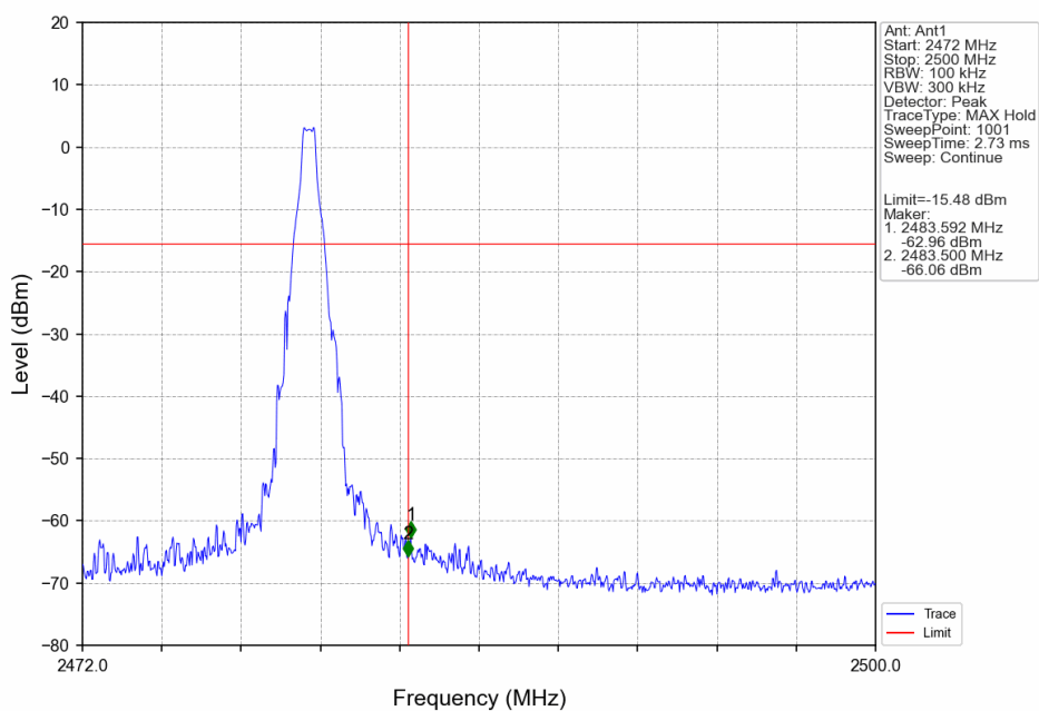
GFSK DH5 HCH 2480MHz_Ant1_NTNV
