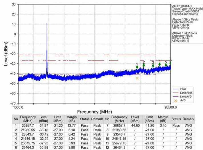
802.11n(HT40)_HCH_5795MHz_Ant1_NTNV
