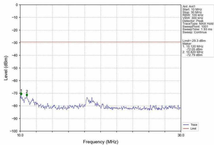
2M_MCH_2440MHz_Ant1_NTNV
