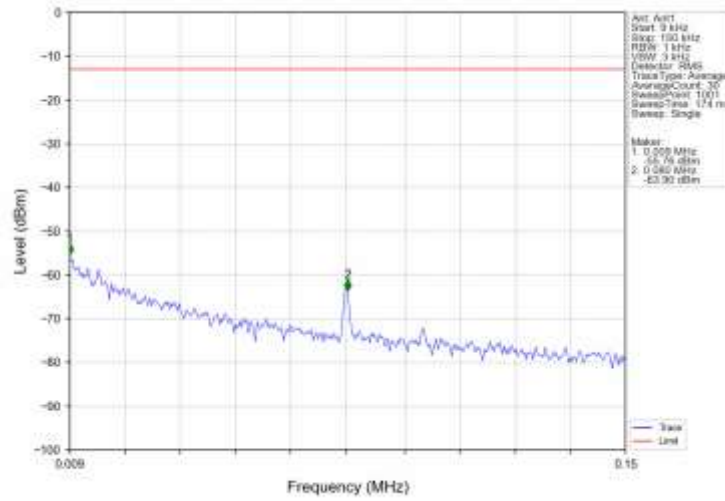
Band17_10MHz_QPSK_MCH_710MHz_RB_1_0_NTNV
