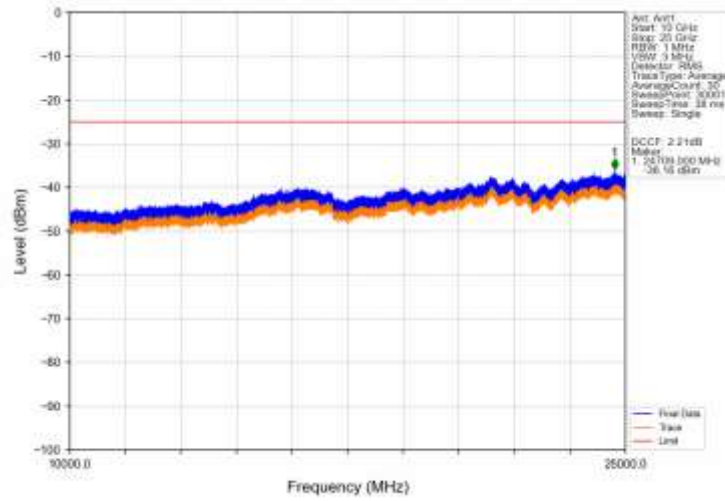
Band41_10MHz_QPSK_HCH_2685MHz_RB_1_0_NTNV
