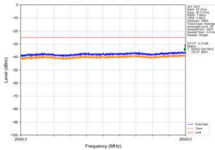
Band41_15MHz_QPSK_MCH_2593MHz_RB_1_0_NTNV
