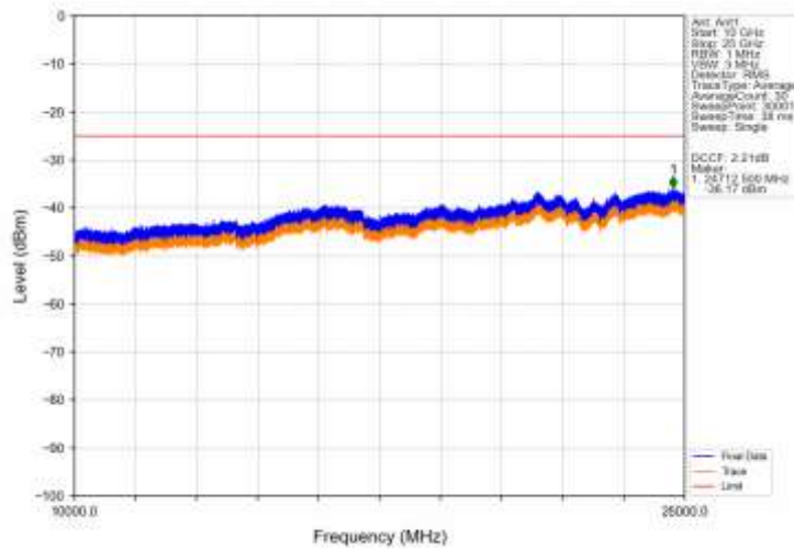
Band41_5MHz_QPSK_LCH_2498.5MHz_RB_1_0_NTNV
