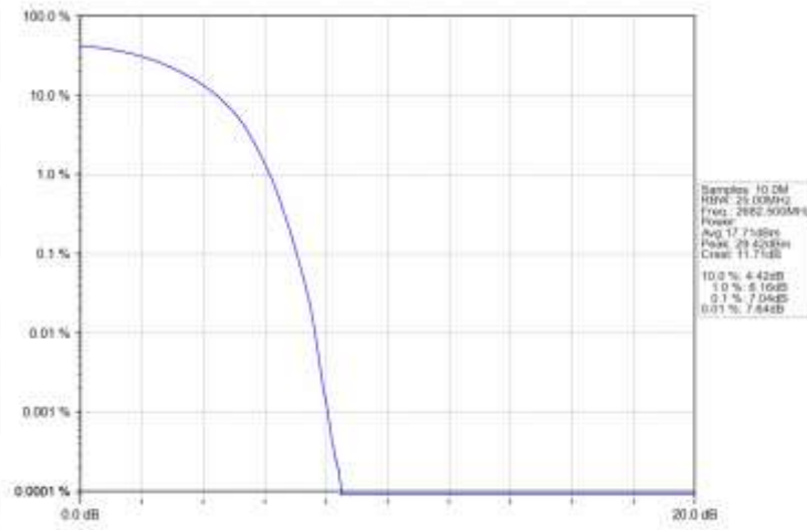
Band41_15MHz_QPSK_HCH_2682.5MHz_RB_75_0_NTNV
