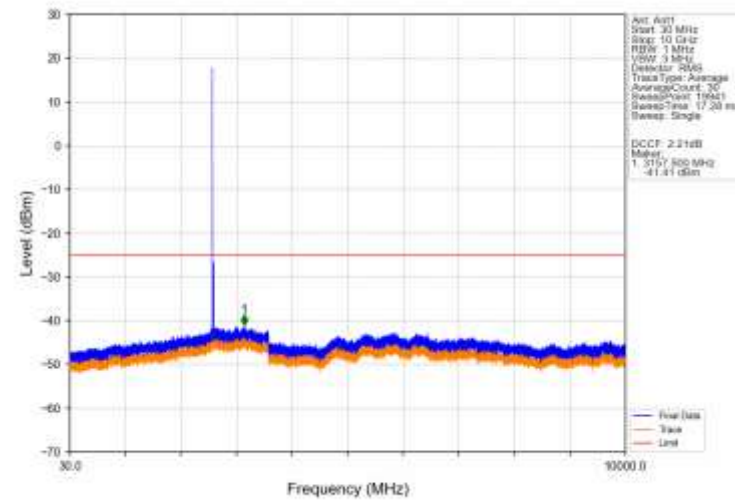
Band41_10MHz_16QAM_MCH_2593MHz_RB_1_0_NTNV
