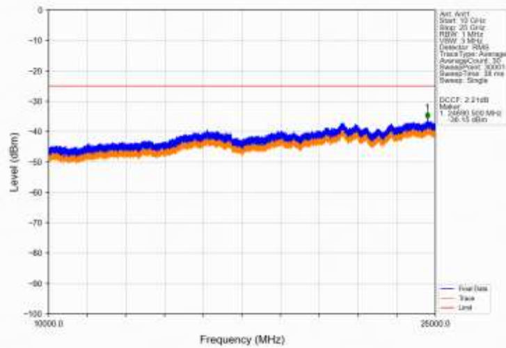
Band41_10MHz_QPSK_MCH_2593MHz_RB_1_0_NTNV
