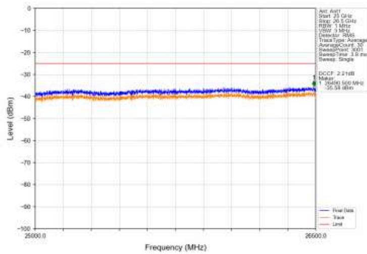
Band41_10MHz_QPSK_MCH_2593MHz_RB_1_0_NTNV
