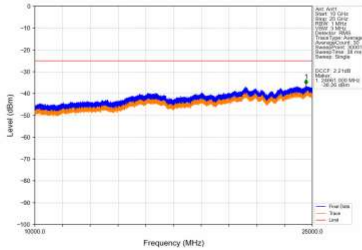
Band41_15MHz_QPSK_MCH_2593MHz_RB_1_0_NTNV
