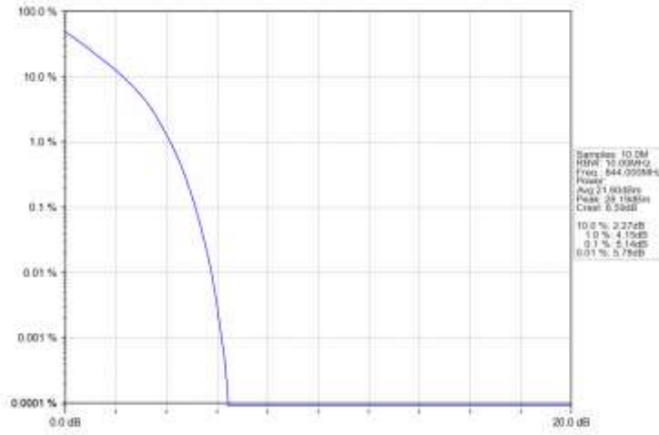
Band5_10MHz_QPSK_HCH_844MHz_RB_50_0_NTNV
