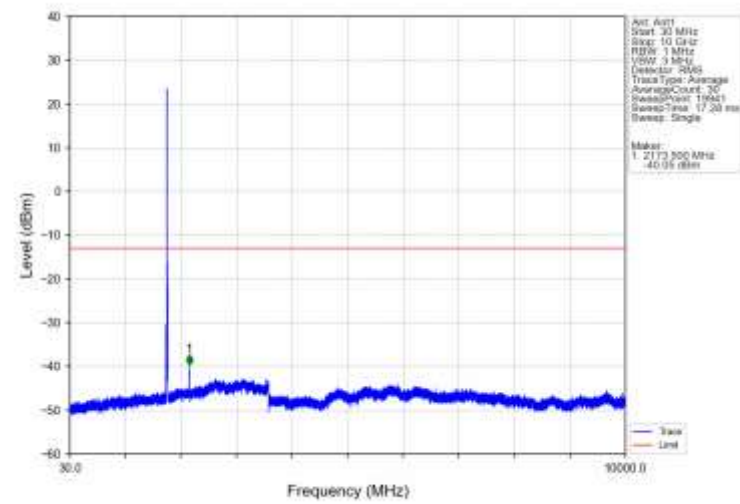
Band66 10MHz QPSK HCH 1775MHz RB 1 0 NTNV
