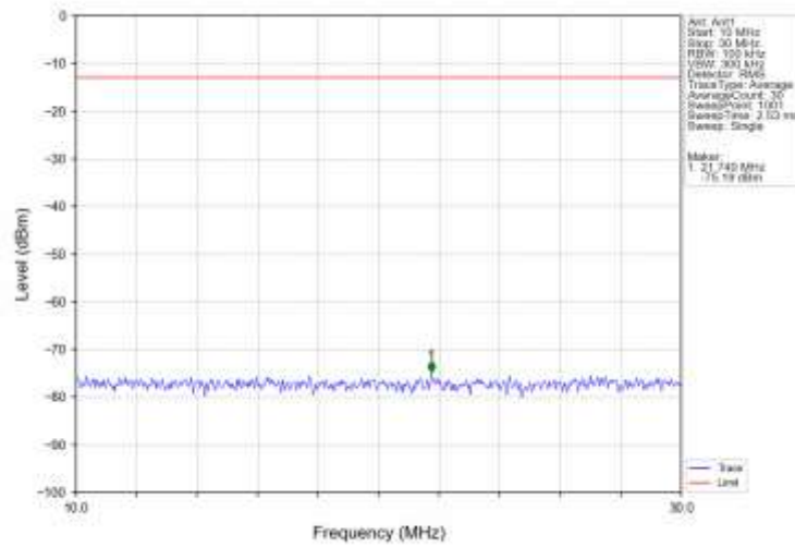
Band66 1.4MHz QPSK LCH 1710.7MHz RB 1 0 NTNV
