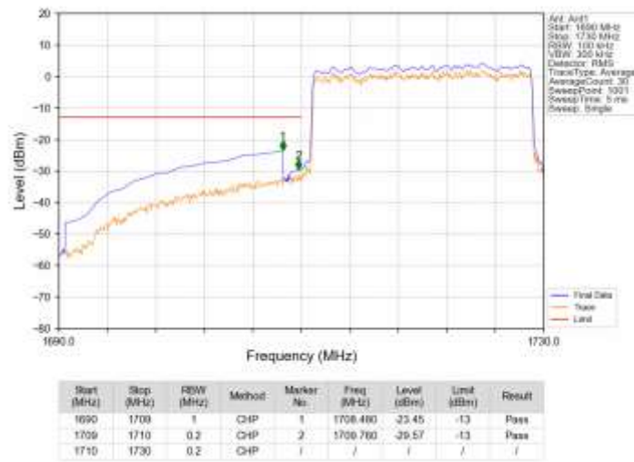
Band66_20MHz_16QAM_LCH_1720MHz_RB_100_0_NTNV
