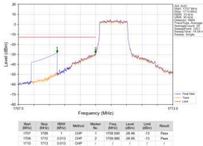
Band66 1.4MHz 16QAM LCH 1710.7MHz RB 6 0 NTNV
