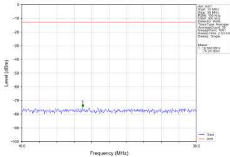
Band66 10MHz QPSK HCH 1775MHz RB 1 0 NTNV
