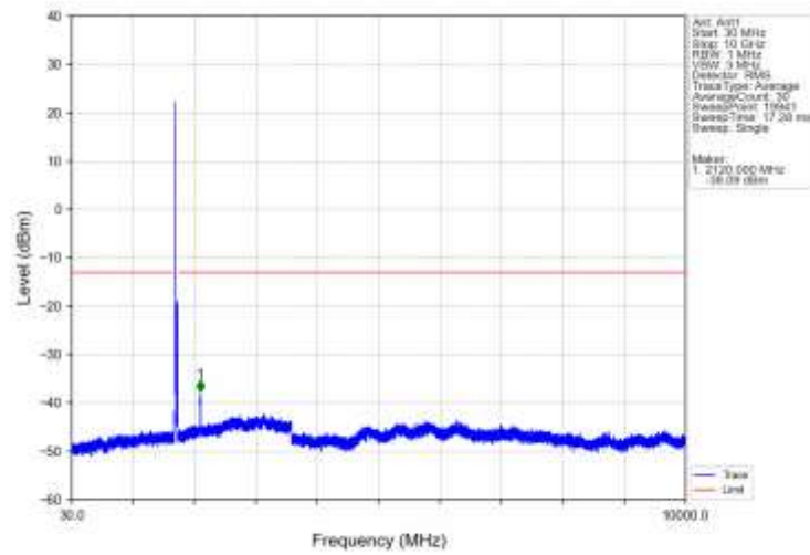
Band66_20MHz_16QAM_LCH_1720MHz_RB_1_0_NTNV
