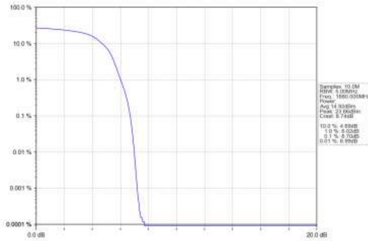
Band2_HSUPA_MCH_1880MHz_Subtest 1_NTNV
