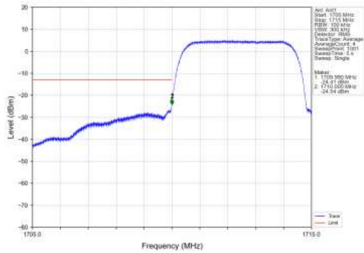
Band4_HSUPA_LCH_1712.4MHz_Subtest 1_NTNV
