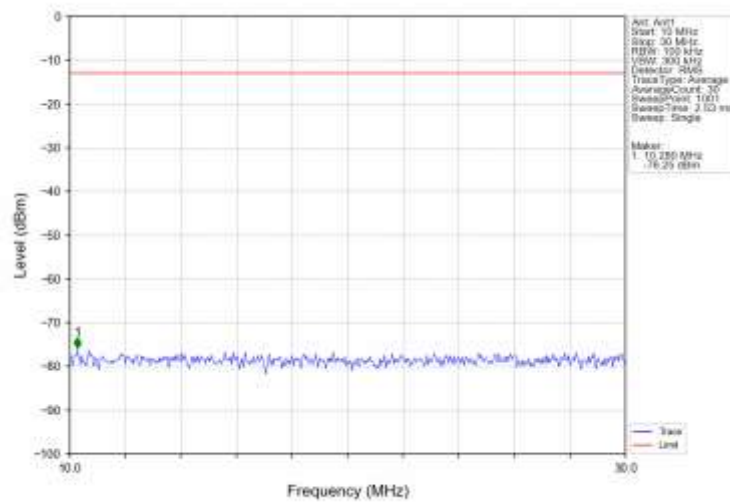
Band4_HSUPA_LCH_1712.4MHz_Subtest 1_NTNV
