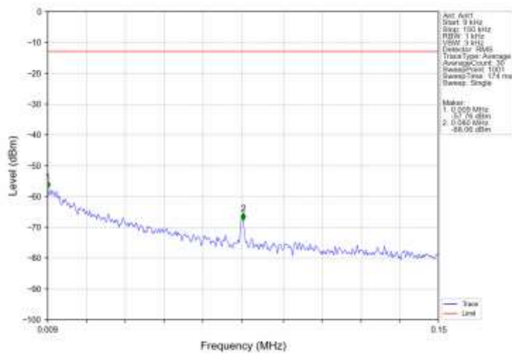
Band5_HSUPA_MCH_836.6MHz_Subtest 1_NTNV
