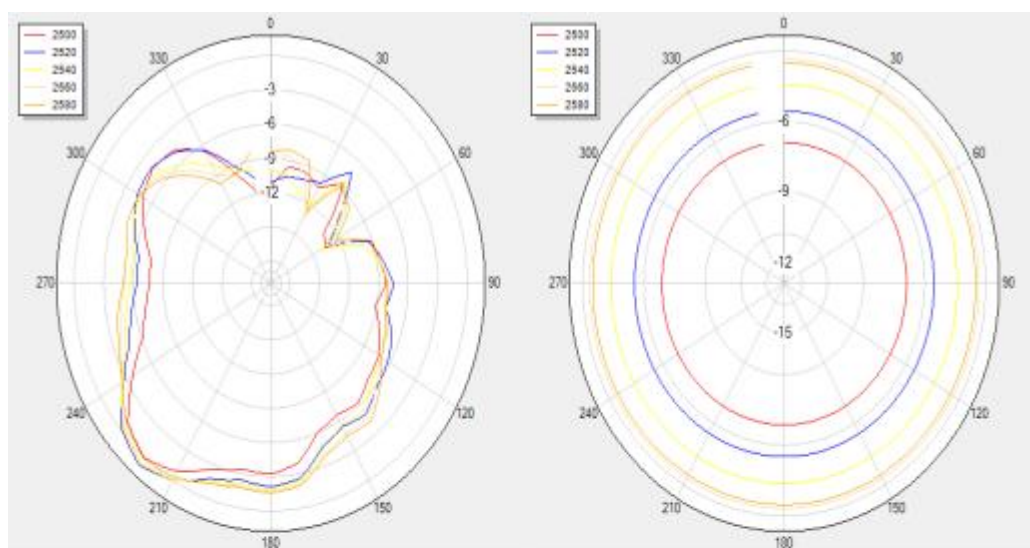
H Theta=90
