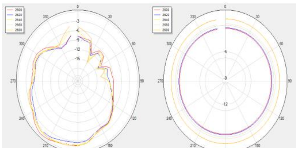
H Theta=90
