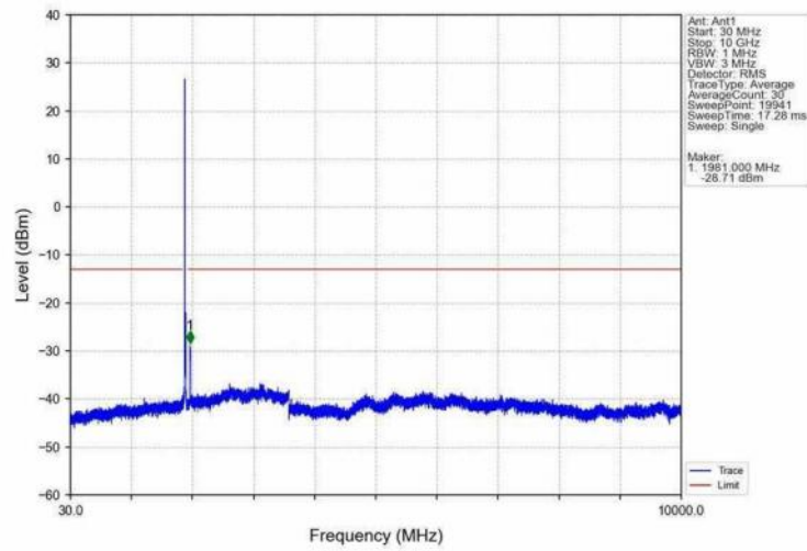
Band25_20MHz_QPSK_HCH_1905MHz_RB_1_0_NTNV
