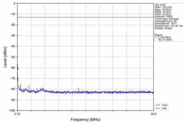
Band25_10MHz_QPSK_HCH_1910MHz_RB_1_0_NTNV
