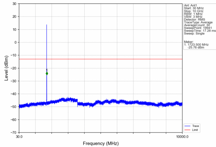
Band4 HSUPA LCH 1712.4MHz Subtest 1 NTNV
