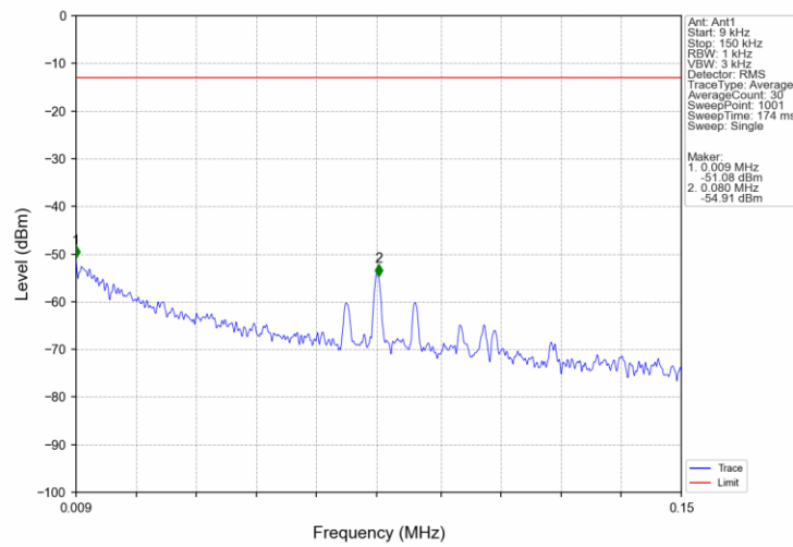
Band4_HSUPA_LCH_1712.4MHz_Subtest 1_NTNV
