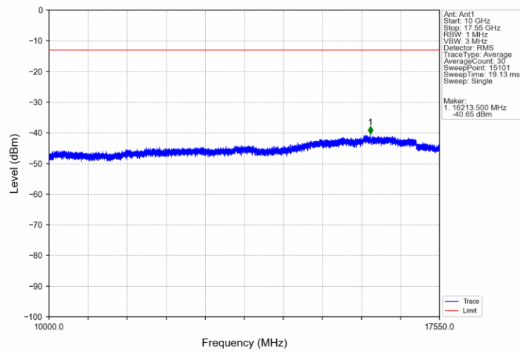
Band4 HSUPA LCH 1712.4MHz Subtest 1 NTNV
