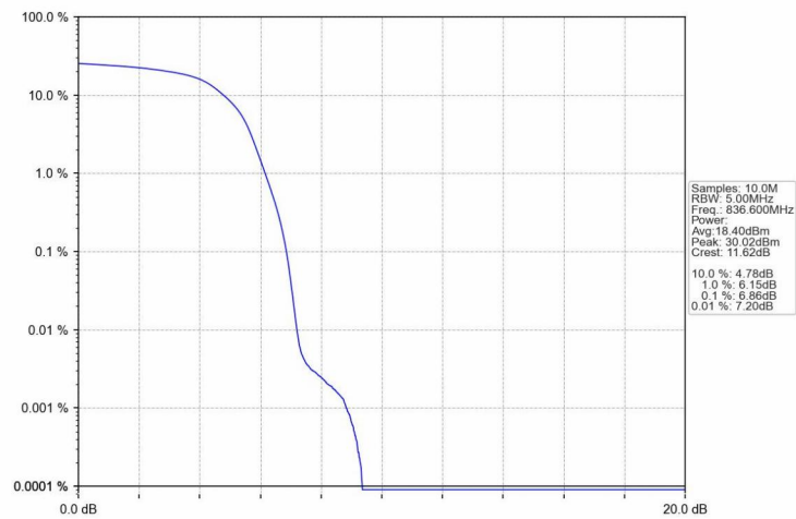
Band5_HSUPA_MCH_836.6MHz_Subtest 1_NTNV
