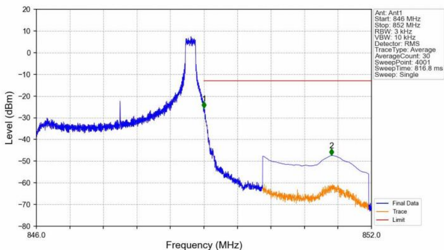
Band5_3MHz_QPSK_HCH_847.5MHz_RB_1_14_NTNV
