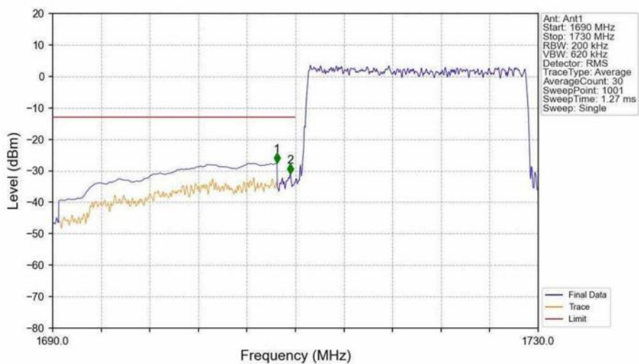
Band66_20MHz_16QAM_LCH_1720MHz_RB_100_0_NTNV
