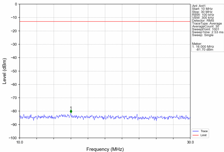
Band4 HSUPA LCH 1712.4MHz Subtest 1 NTV
