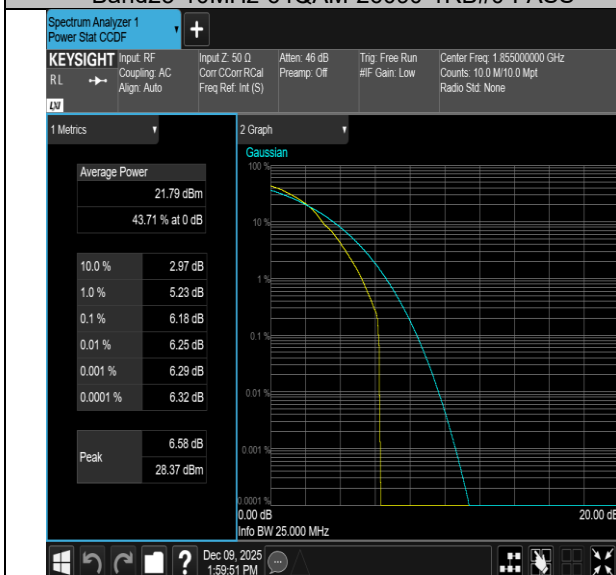
Band25-10MHz-64QAM-26365-1RB#0-PASS
