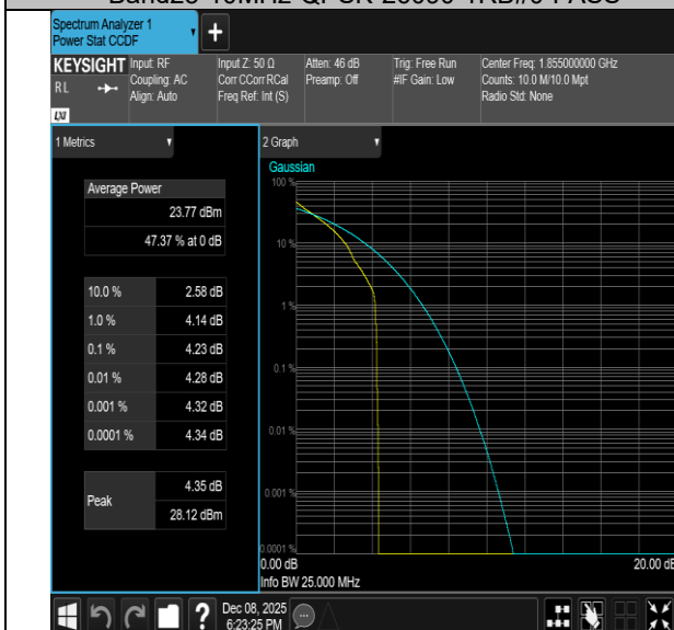
Band25-10MHz-QPSK-26365-1RB#0-PASS
