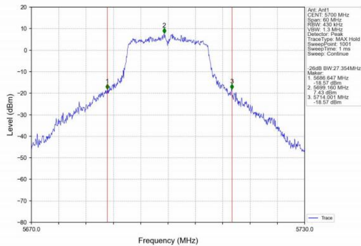
802.11n(HT20)_HCH_5700MHz_Ant1_NTNV
