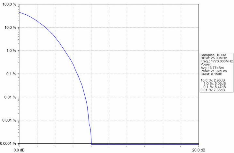
n66_30kHz_SISO_NTNV_20MHz_DFT-s-OFDM_256_QAM_1770MHz_Outer_Full_Ant1
