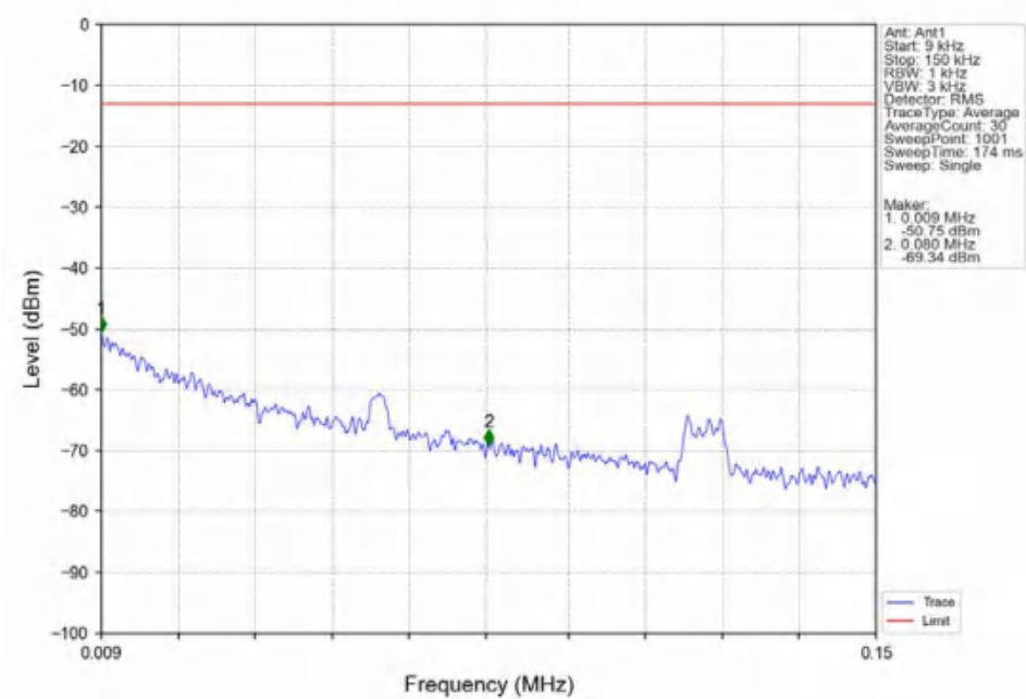
Band2_3MHz_QPSK_MCH_1880MHz_RB_1_0_NTNV
