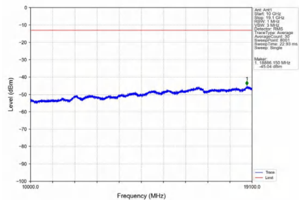
Band2_10MHz_16QAM_LCH_1855MHz_RB_50_0_NTNV
