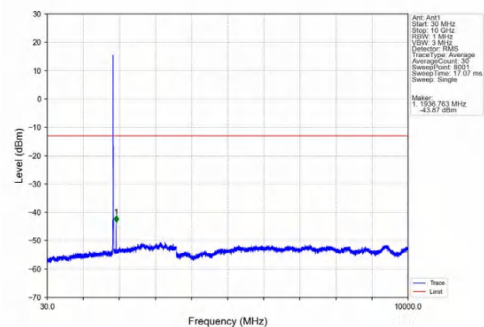
Band2_10MHz_16QAM_LCH_1855MHz_RB_1_0_NTNV
