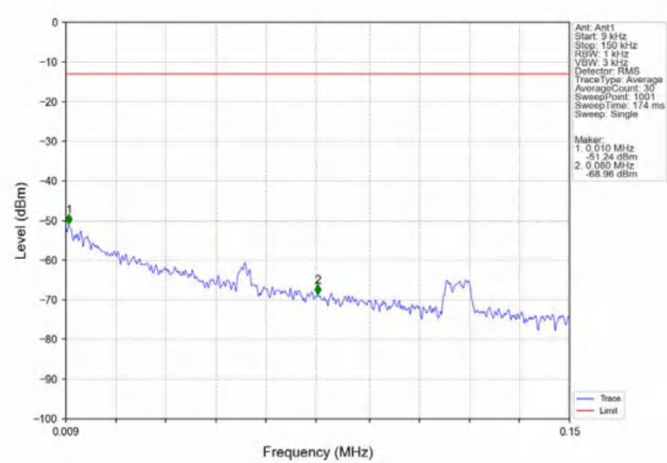
Band2_10MHz_QPSK_MCH_1880MHz_RB_1_0_NTNV
