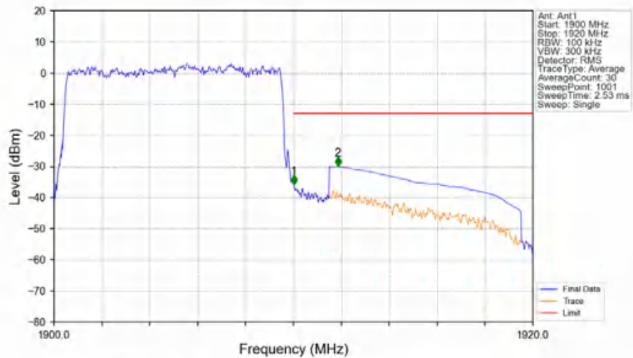
Band2_10MHz_QPSK_HCH_1905MHz_RB_50_0_NTNV
