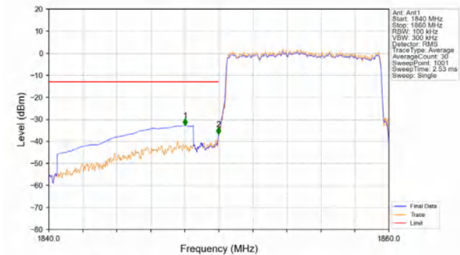
Band2_10MHz_16QAM_LCH_1855MHz_RB_50_0_NTNV
