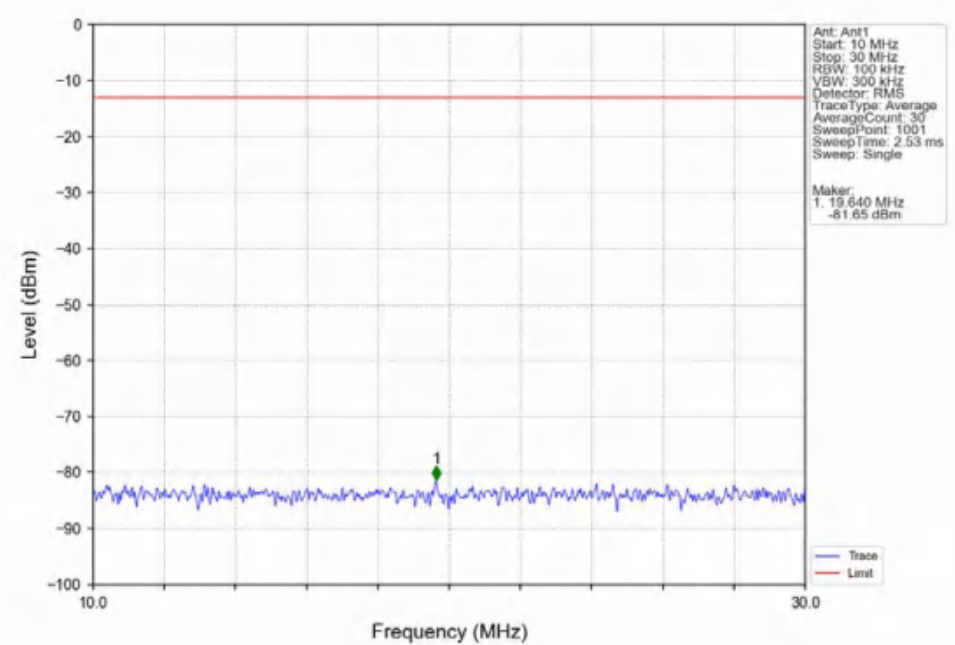
Band2_10MHz_16QAM_LCH_1855MHz_RB_1_0_NTNV
