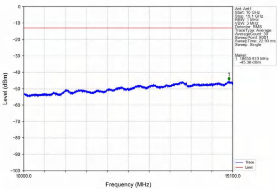
Band2_5MHz_QPSK_MCH_1880MHz_RB_1_0_NTNV
