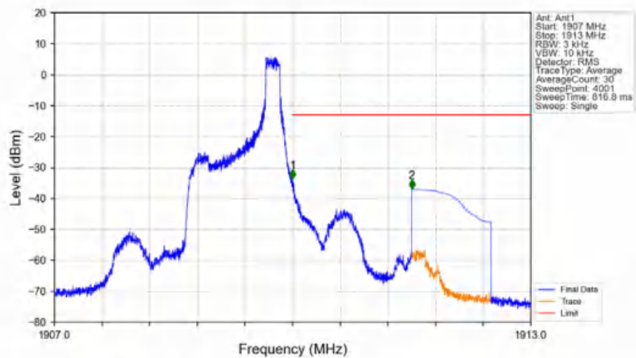
Band2_1.4MHz_QPSK_HCH_1909.3MHz_RB_1_5_NTNV
