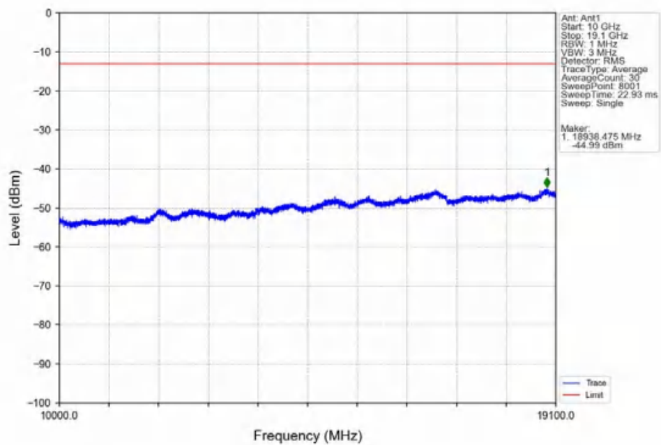
Band2_1.4MHz_QPSK_HCH_1909.3MHz_RB_1_5_NTNV
