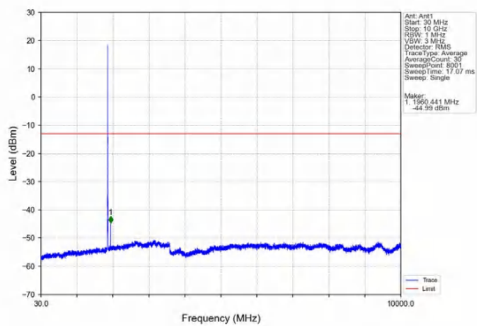
Band2_5MHz_QPSK_MCH_1880MHz_RB_1_0_NTNV
