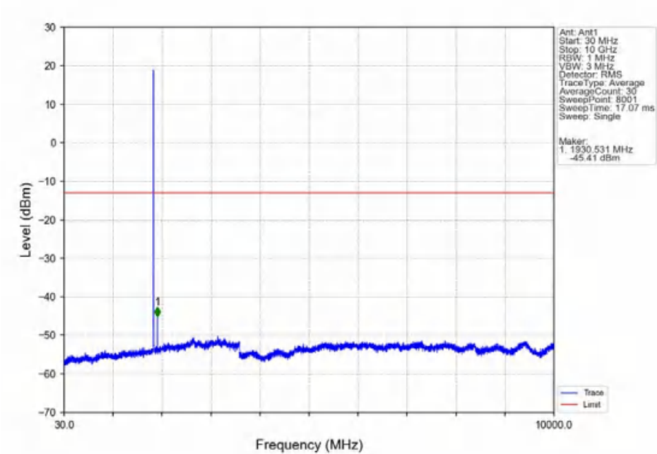
Band2_3MHz_QPSK_LCH_1851.5MHz_RB_1_0_NTNV
