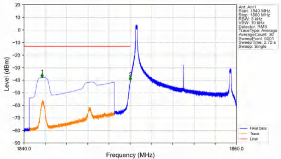
Band2_10MHz_16QAM_LCH_1855MHz_RB_1_0_NTNV
