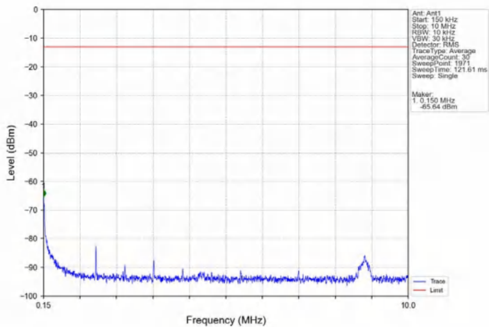
Band2_10MHz_16QAM_MCH_1880MHz_RB_1_0_NTNV
