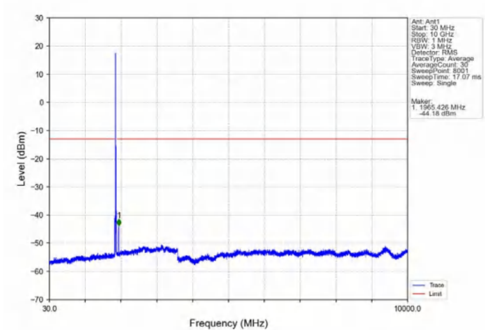
Band2_15MHz_QPSK_MCH_1880MHz_RB_1_0_NTNV
