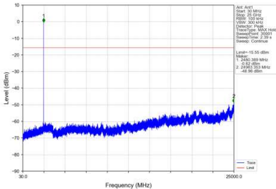
Pi/4DQPSK 2DH5 HCH 2480MHz Ant1 NTV
