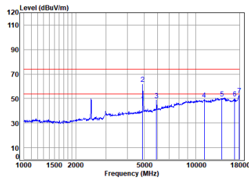
11g_TX_CH_11_Horizontal
