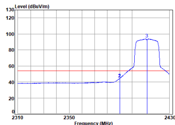
11n_HT(20M)_TX_CH_01_Vertical-Avg
