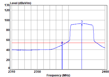
11n_HT(40M)_TX_CH_03_Horizontal-Avg
