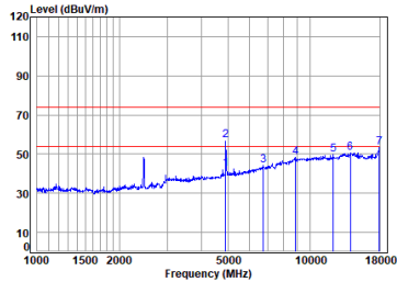
11n_20M_TX_CH_11_Horizontal
