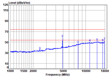
11ax_20M_TX_CH_11_Horizontal
