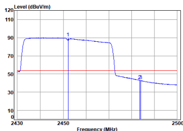
11ax_40M_TX_CH_09_Vertical-Avg
