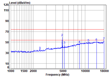
11ax_20M_TX_CH_11_Vertical
