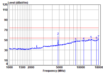
11ax_20M_TX_CH_01_Horizontal
