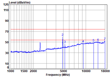
11n_20M_TX_CH_11_Vertical
