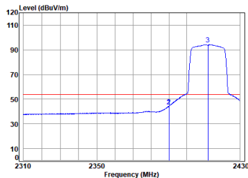
11ax_20M_TX_CH_01_Vertical-Avg
