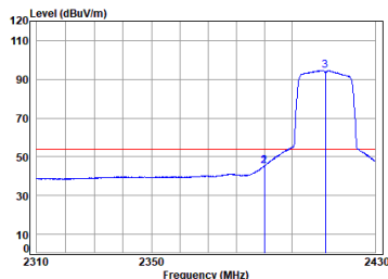
11ax_20M_TX_CH_01_Horizontal-Avg
