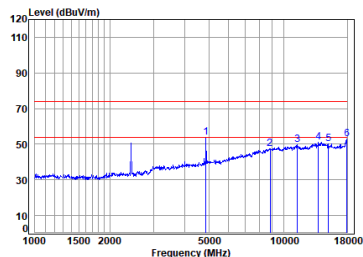
11b_TX_CH_06_Horizontal
