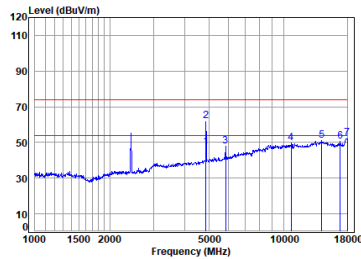
11g_TX_CH_06_Horizontal
