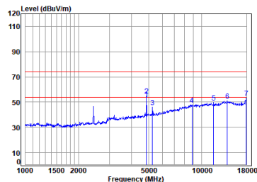
11b_TX_CH_06_Vertical
