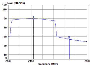
11ax_40M_TX_CH_09_Horizontal-Avg
