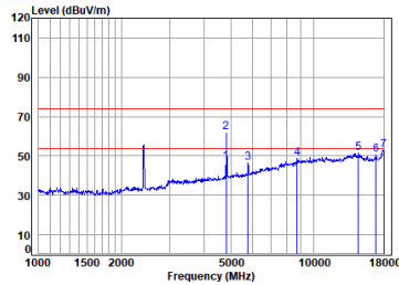
11g_TX_CH_01_Horizontal
