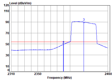
11ax_40M_TX_CH_03_Horizontal-Avg
