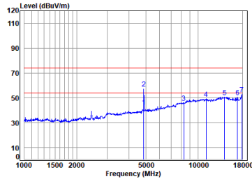
11ax_20M_TX_CH_06_Horizontal
